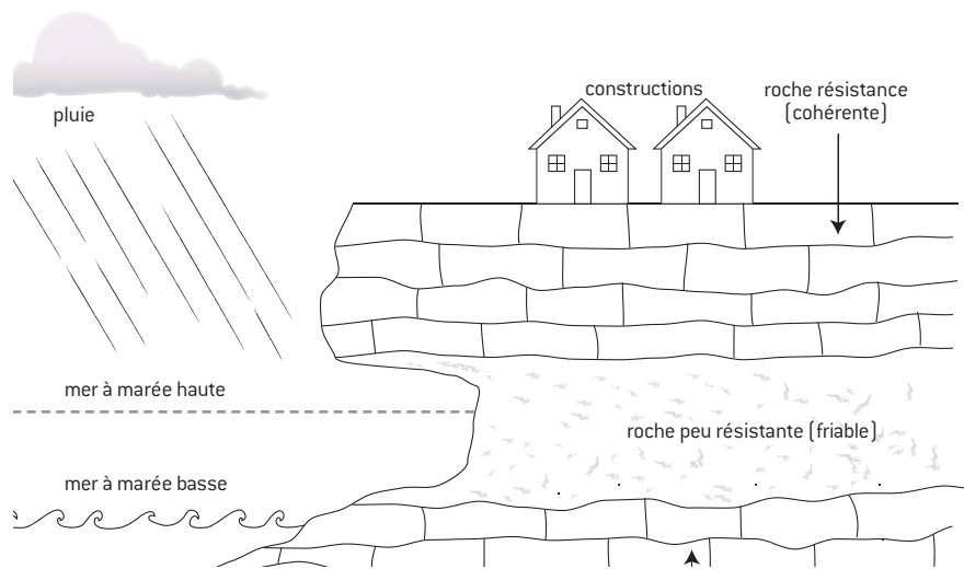
Doc. 1. Schéma simplifié d'un affleurement en bord de mer
